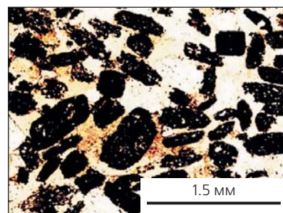
Рис.13. Неясно-слоистая богатая ярегская лейкоксовая руда состава (%): \text{SiO}_2 — 32.65, \text{Al}_2\text{O}_3 — 4.64, \text{TiO}_2 — 31.78, \text{Fe}_2\text{O}_3 — 15.75, \text{MnO} — 0.30, \text{MgO} — 0.81, \text{CaO} — 0.81, \text{Na}_2\text{O} — 0.61, \text{K}_2\text{O} — 1.43, \text{P}_2\text{O}_5 — 0.20, потери при прокаливании — 11.0, Ва — 0.008; сумма — 99.98. Слева — сканограмма образца, справа — шлиф, николи параллельны. Черное — лейкоксен.
