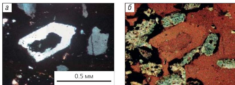
Рис.8. Футляровидный кристалл кварца в лейкоксеновой руде. Шлиф 17–22: а — николи скрещены, б — в косом свете. Серые зерна — лейкоксен.
