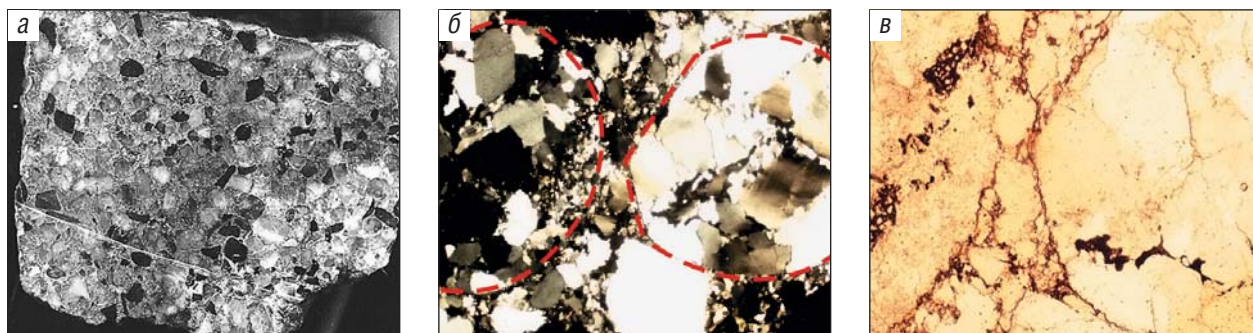
Рис. 5. Гравелитоподобный метасоматит (образец ПАЧ-АН): а — сканограмма пришлифовки, б — шлиф, николи скрещены; в — деталь того же шлифа с реликтами замещающей породы в метасоматических шариках, николи параллельны.
