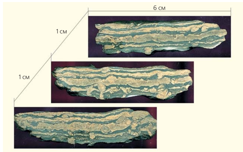
Рис.10. Новообразованная (флюидотурбитная) псевдослойчатость в Чибьюской субформации. Ярегская нефтяная шахта №3. Блок-диаграмма из сканограмм трех шлифованных срезов с шагом 1 см.
