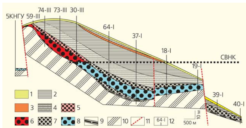
Рис.6. Строение Чибьюской титановорудной субформации (по материалам Ярегского нефтешахтоуправления). 1 — титановорудные конгломераты и песчаники нижнефранской субформации, 2–9 — породы и руды: 2 — аргиллиты третьей пачки, 3 — лейкоксеновые руды третьей пачки, 4 — аргиллиты и алевролиты второй пачки (надрудные алевролиты) с линзами лейкоксеновых руд, 5 — нефтенасыщенные бедные лейкоксеновые руды второй пачки, 6 — нефтенасыщенные богатые лейкоксеновые руды второй пачки, 7 — бедные лейкоксеновые руды второй пачки без нефти, 8 — богатые лейкоксеновые руды второй пачки без нефти, 9 — «надсланцевые аргиллиты» первой пачки; 10 — рифей-вендские сланцы, 11 — разломы, 12 — скважины. СВНК — современный водонефтяной контакт.
