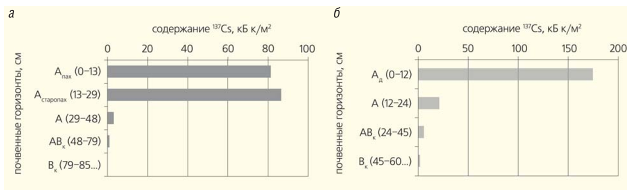
Рис.5. Профильное распределение запасов ^{137}\text{Cs} в пахотных (а) и целинных (б) черноземах Плавского радиоактивного пятна. Черноземы сформированы на карбонатных (содержащих карбонаты кальция) лессовидных суглинках. Обозначения горизонтов почв: А — гумусовый; А пах — пахотный; А старопах — старопахотный; А д — дерновый; В к — иллювиальный карбонатный горизонт; АВ к — переходный горизонт от гумусового к иллювиальному, карбонатный.
