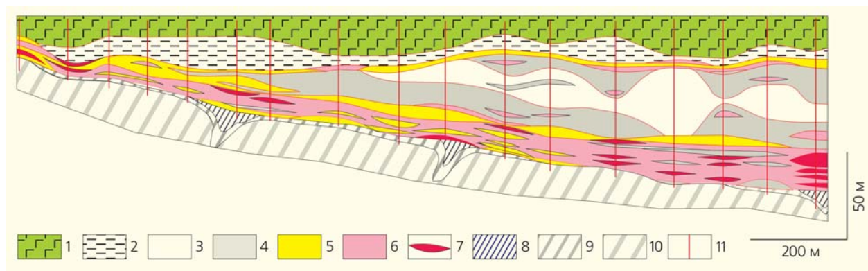
Рис. 4. Распределение TiO_2 в титаноносной формации и в подстилающих вендских сланцах (использованы материалы Ярегского нефтешахтоуправления). 1 — вулканогенно-осадочная субформация, 2 — аргиллиты нижнефранской субформации, 3–7 — концентрации TiO_2 : 3 — менее 1%, 4 — 1–2.5%, 5 — 2.5–7%, 6 — 7–15%, 7 — более 15%; 8–10 — вендские сланцы с концентрациями TiO_2 : 8 — 1–2.6%, 9 — 0.7–1%, 10 — менее 0.7%; 11 — разведочные скважины.
