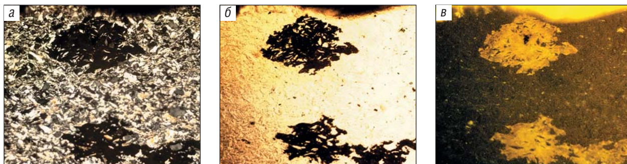
Рис.12. Ситовидная структура метасоматических кристаллобластов лейкоксена в аргиллите надвулканогенной титановорудной субформации. Шлиф 17–72: а — николи скрещены, б — николи параллельны, в — в косом свете.
