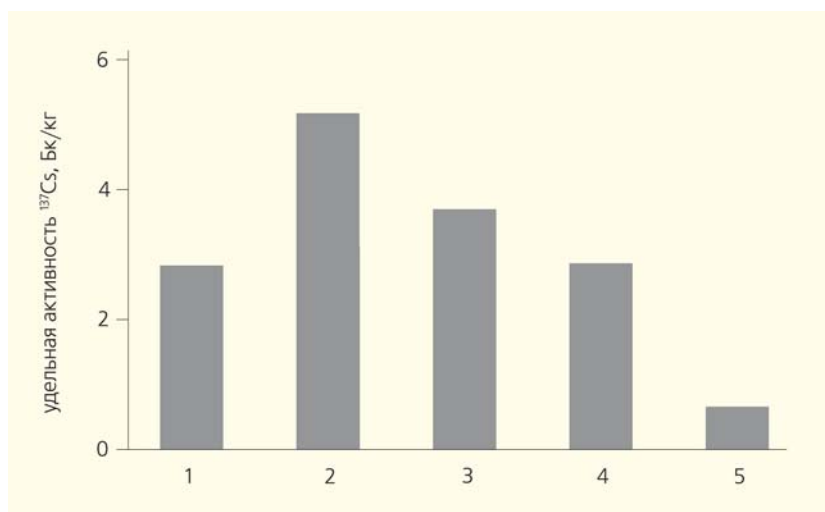
Рис.7. Удельная активность ^{137}\text{Cs} (Бк/кг) в различных фракциях биомассы клубней картофеля, выращенного на территории Плавского радиоактивного пятна: 1 — очистка, 2 — центральная часть клубня, 3 — сок, 4 — крахмалистый осадок, 5 — жмых.
