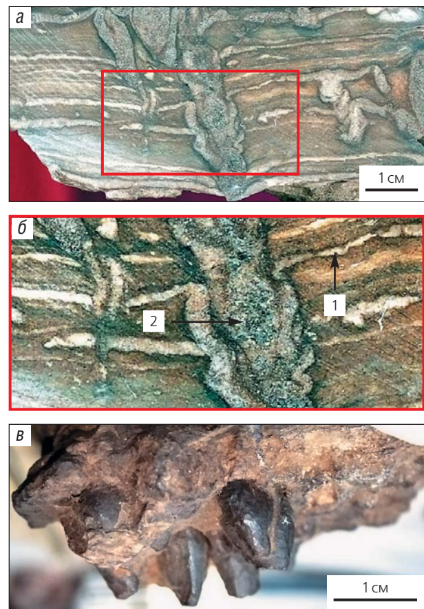
Рис.11. Лейкоксен-кварцевые морфогенетические аналоги структуры конус-в-конусе. Детали флюидотурбитной текстуры в Чибьюской субформации: а — сканограмма шлифованного образца Я-22; б — деталь сканограммы (стрелками показан лейкоксен-кварцевый след: 1 — полойно проникающего флюида, 2 — пронизывающего слоистость), в — фото того же образца с препарированными конусами. Нефтяная шахта №3.
