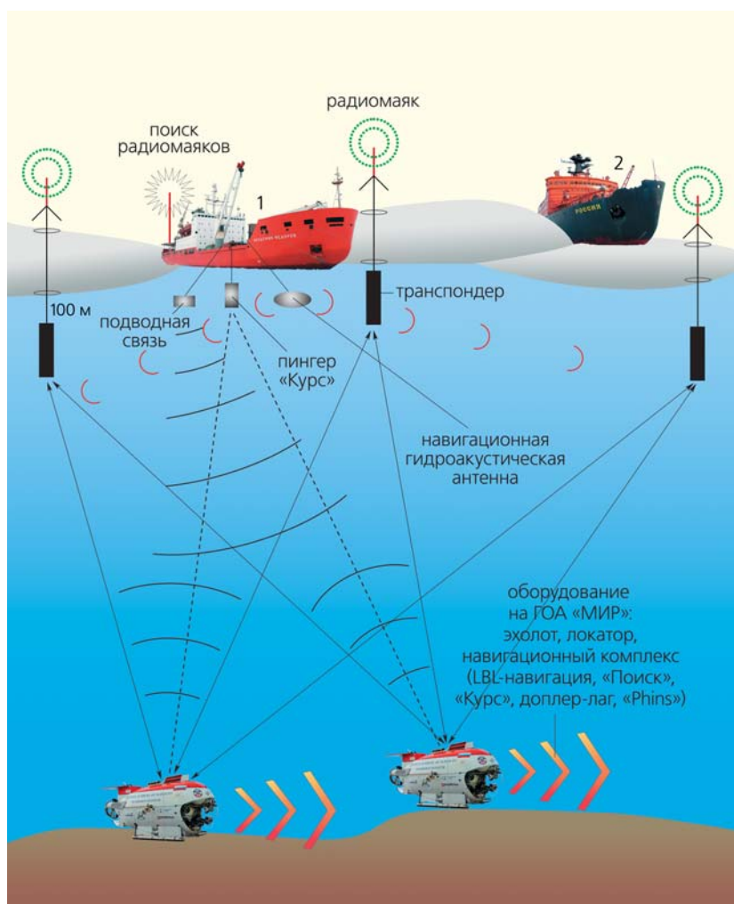
Система гидроакустической навигации, применявшаяся при погружении «Миров» на Северном полюсе. 1 — НИС «Академик Федоров», 2 — атомный ледокол «Россия».
