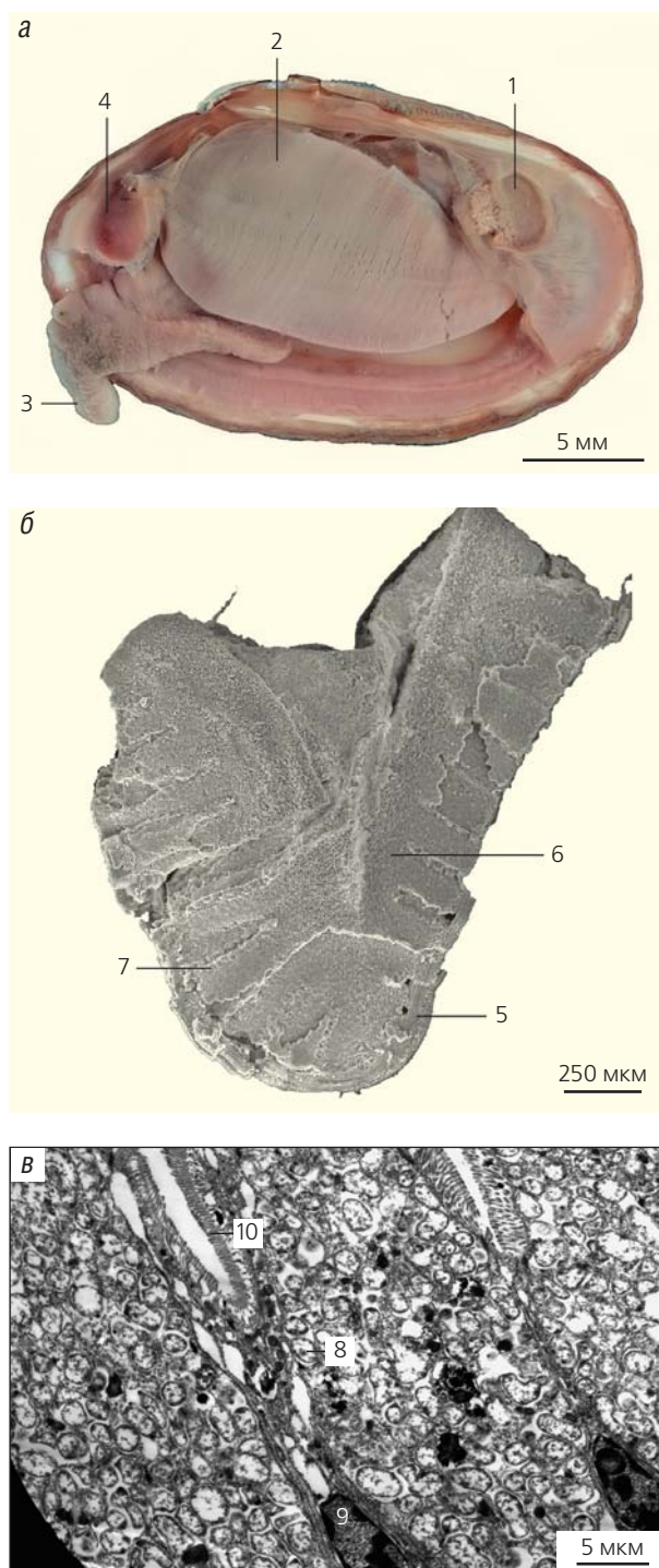
Рис.2. Строение плиокардиины: а — тело Calyplogena pacifica (левая створка удалена), 1 — задний мускул-замыкатель, 2 — левая жабра, 3 — нога, 4 — передний мускул-замыкатель; б — внутреннее строение жабры (сканирующий электронный микроскоп), 5 — жаберный филламент; 6 — септа, состоящая из бактериоцитов и заполняющая пространство между филламентами, 7 — отдельные бактериоциты, различаемые в септе; в — жаберный эпителий плиокардиины, в котором видны специализированные клетки бактериоциты, содержащие многочисленные бактерии, и узкие промежуточные клетки с ядрами у основания бактериоцитов (просвечивающий электронный микроскоп), 8 — бактерии, 9 — ядро, 10 — микровилли.
