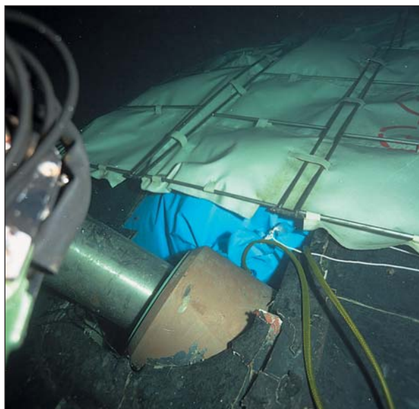
Работа ГОА «Мир» на атомной подводной лодке «Комсомолец»: введение гамма-спектрометра в вентиляционную трубу реактора атомной лодки (слева), герметизация ее носовой части (справа).
