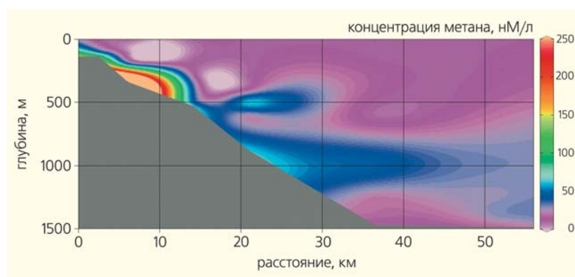
Рис.4. Диаграмма распределения метана в морской воде на профиле 4.
