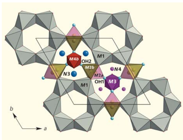
Рис.4. Распределение \text{Fe}^{3+} по M2 -подпозициям в структуре сиудайта в проекции на плоскость (110).
