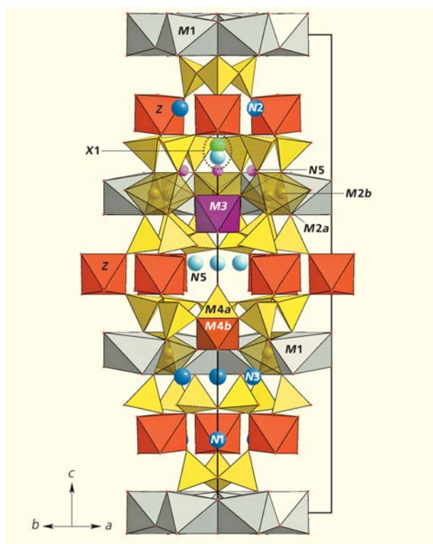
Рис.3. Общий вид структуры сиудайта вдоль длинного параметра ячейки вокруг оси третьего порядка.
