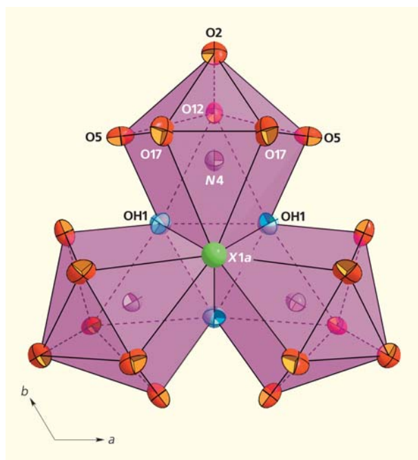
Рис.7. Связь N4 -полиэдров.
