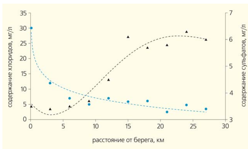
Рис. 1. Точечные диаграммы содержания хлоридов (кружки) и сульфатов (треугольники) в пробах осадков и в озерной воде на Кольском п-ове на разных расстояниях от морского берега. Пунктиром соответствующего цвета показаны линии тренда — логарифмическая для хлоридов и полиномиальная для сульфатов.
